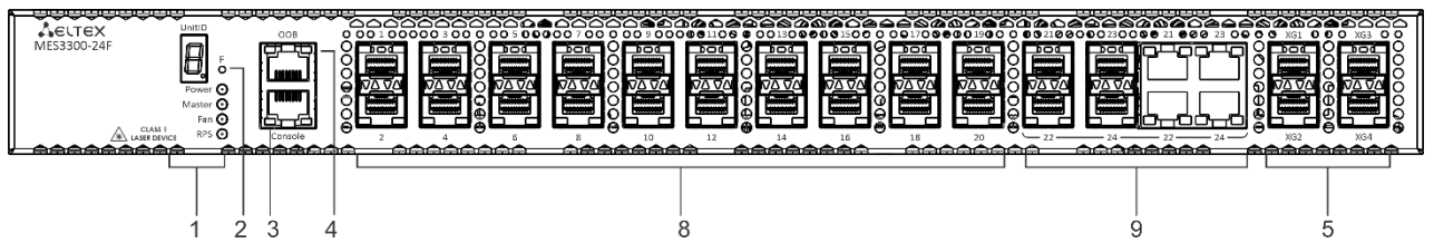
Рисунок 18 – Передняя панель MES3300-24F
