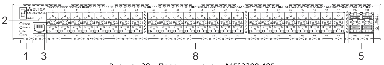
Рисунок 20 – Передняя панель MES3300-48F
