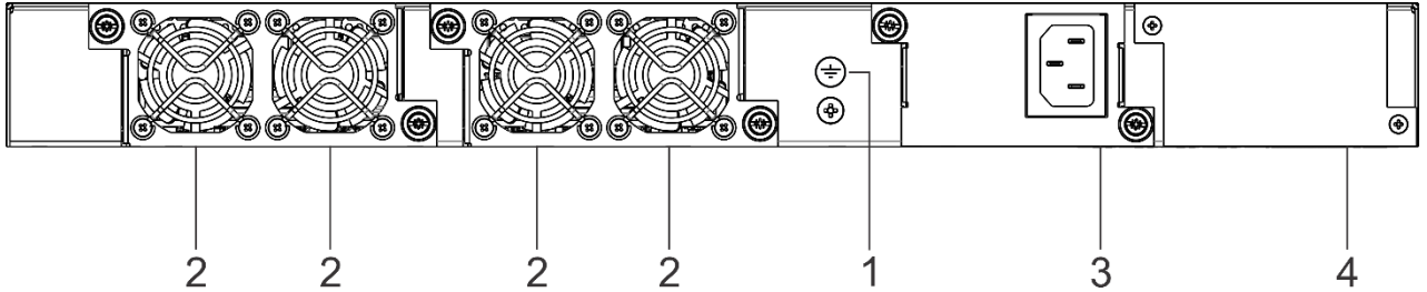
Рисунок 50 – Задняя панель MES3300-24F
