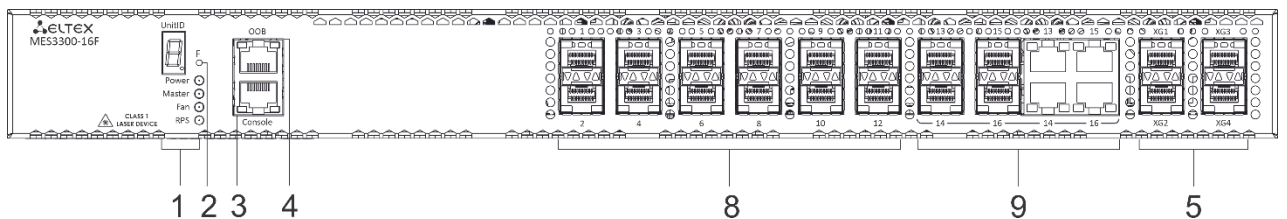
Рисунок 17 – Передняя панель MES3300-16F
