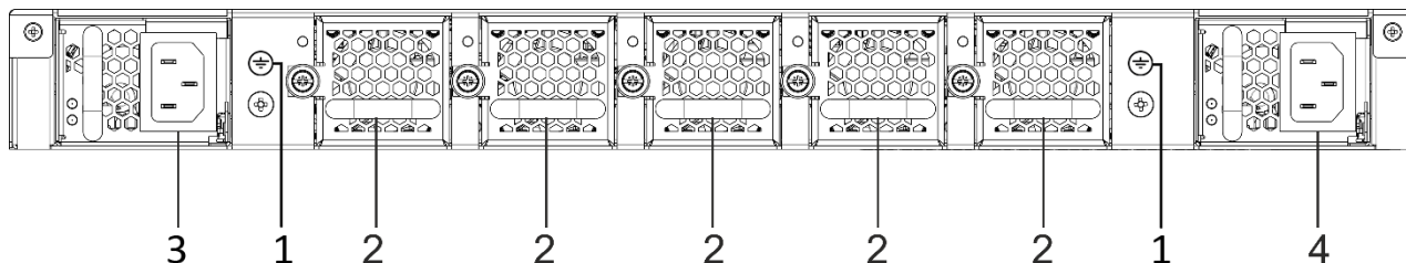
Рисунок 60 – Задняя панель MES5500-32
