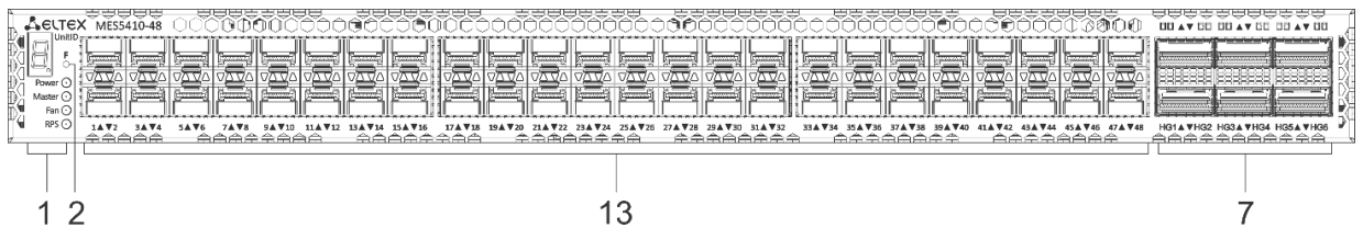
Рисунок 31 – Передняя панель MES5410-48
