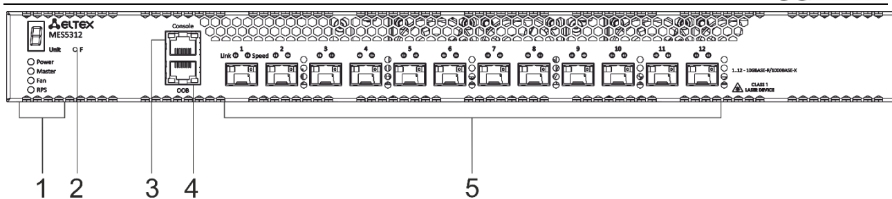
Рисунок 21 – Передняя панель MES5312
