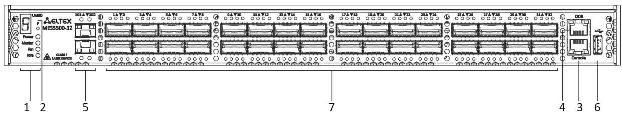
Рисунок 32 – Передняя панель MES5500-32
