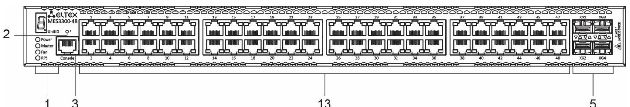
Рисунок 19 – Передняя панель MES3300-48
