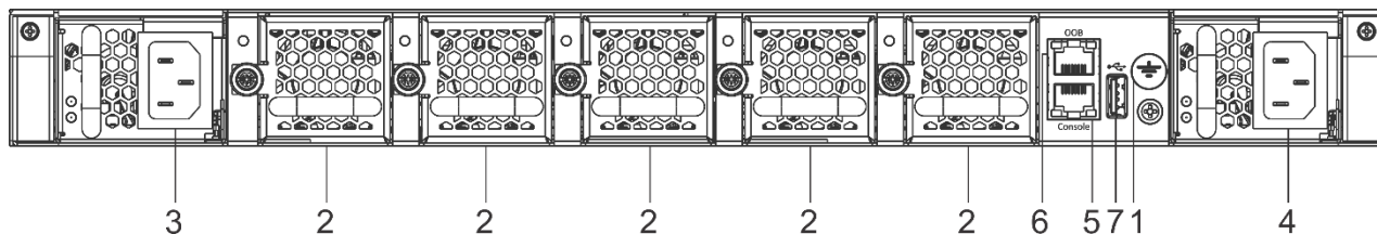
Рисунок 59 – Задняя панель MES5410-48
