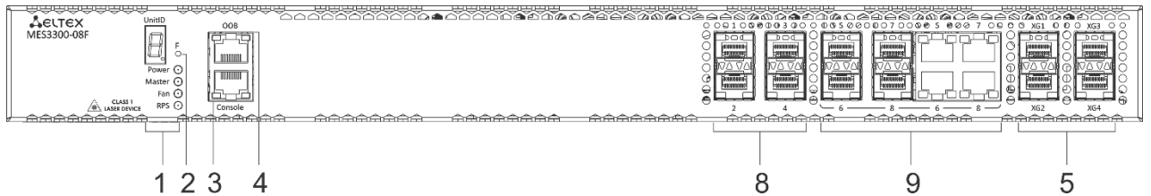
Рисунок 16 – Передняя панель MES3300-08F
