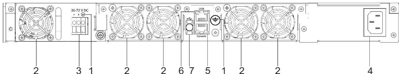
Рисунок 58 – Задняя панель MES5400-48
