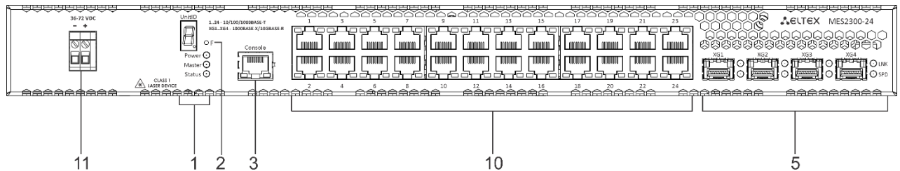
Рисунок 4 – Передняя панель MES2300-24 DC
