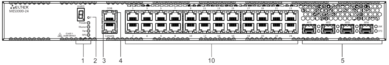
Рисунок 15 – Передняя панель MES3300-24
