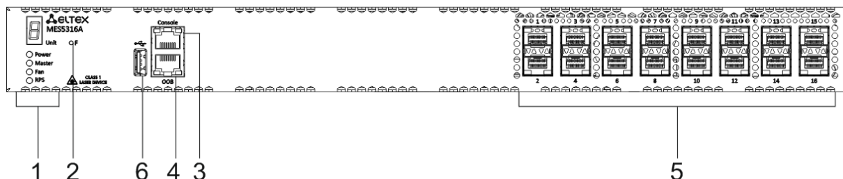
Рисунок 22 – Передняя панель MES5316A
