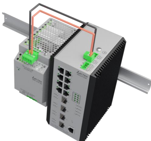
Рисунок 62 – Подключение питания коммутатора от DRS-270-56
