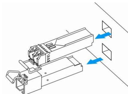
Рисунок 69 – Извлечение SFP-трансиверов
