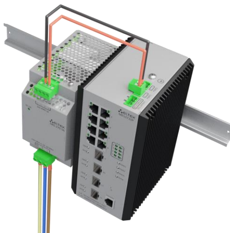
Рисунок 64 — Подключение питания коммутатора от одного блока питания DRS-270-56
