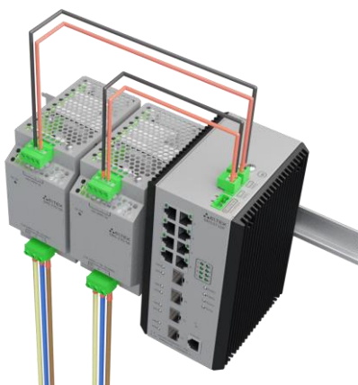
Рисунок 65 — Подключение питания коммутатора от двух блоков питания DRS-270-56
