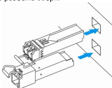
Рисунок 66 – Установка SFP-трансиверов
