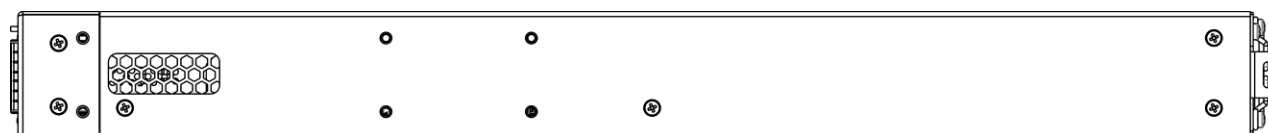
Рисунок 17 – Правая боковая панель Ethernet-коммутатора MES5400-48
