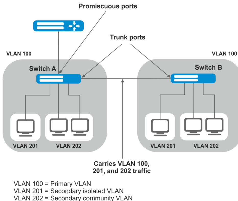
Рисунок 30 – Пример работы технологии Private VLAN
