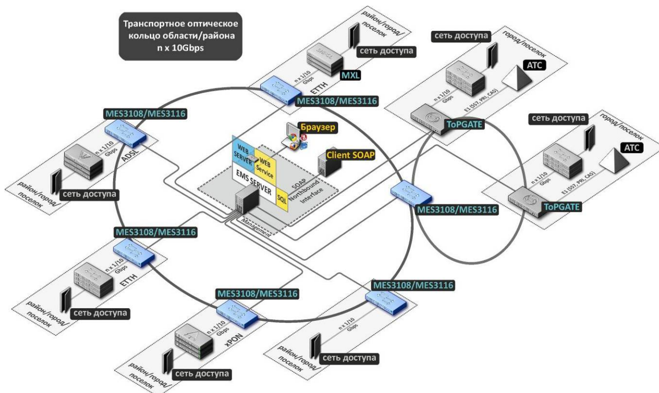
Рисунок 16 – Структура системы управления «Eltex.EMS» для цифровых транспортных систем
