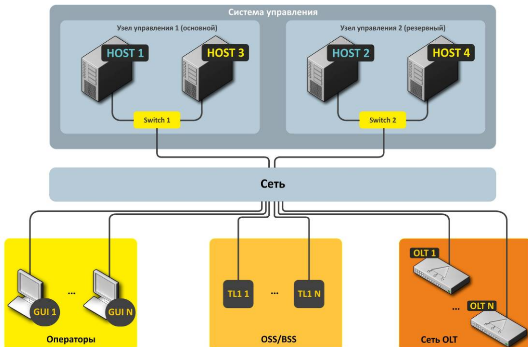
Рисунок 1г — Укрупнённая схема организации связи
