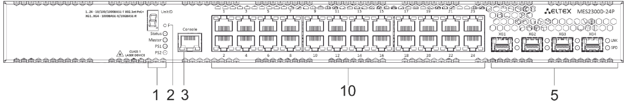
Рисунок 12 – Передняя панель MES2300D-24P
