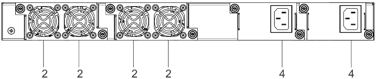
Рисунок 47 – Задняя панель MES3300-24, MES5300-24
