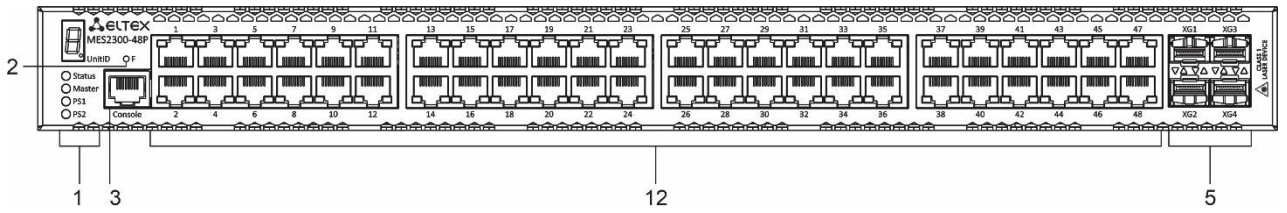
Рисунок 13 – Передняя панель MES2300-48P
