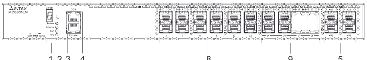
Рисунок 17 – Передняя панель MES3300-16F
