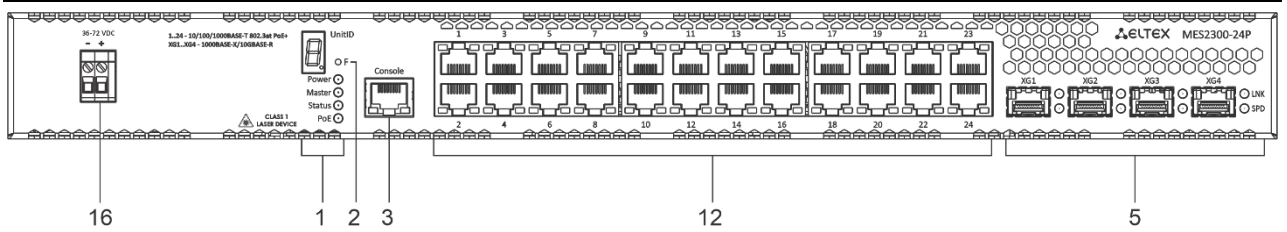
Рисунок 11 – Передняя панель MES2300-24P DC
