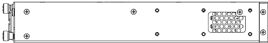
Рисунок 76 – Левая боковая панель MES5316A, MES5324A, MES5332A
