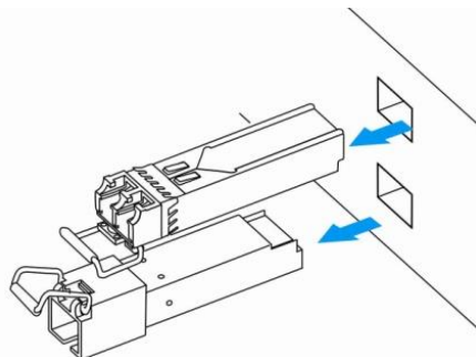
Рисунок 100 – Извлечение SFP-трансиверов
