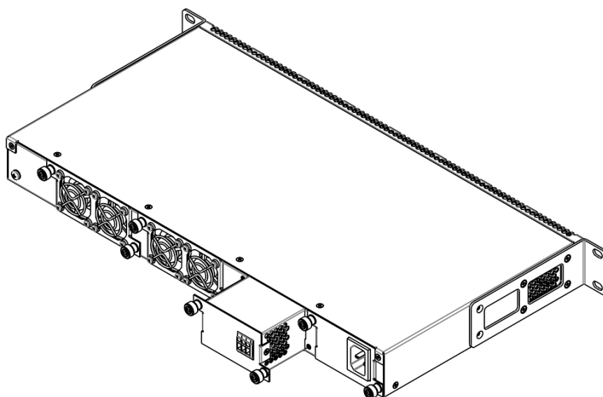
Рисунок 96 – Установка модулей питания
