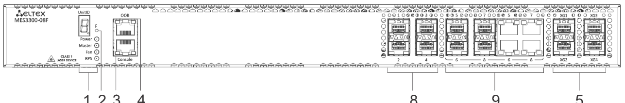
Рисунок 16 – Передняя панель MES3300-08F
