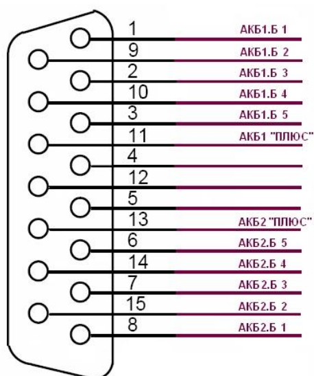
разъем Battery Sense
