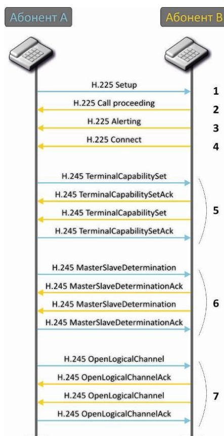
Рисунок 24 – Алгоритм вызова по протоколу H.323
