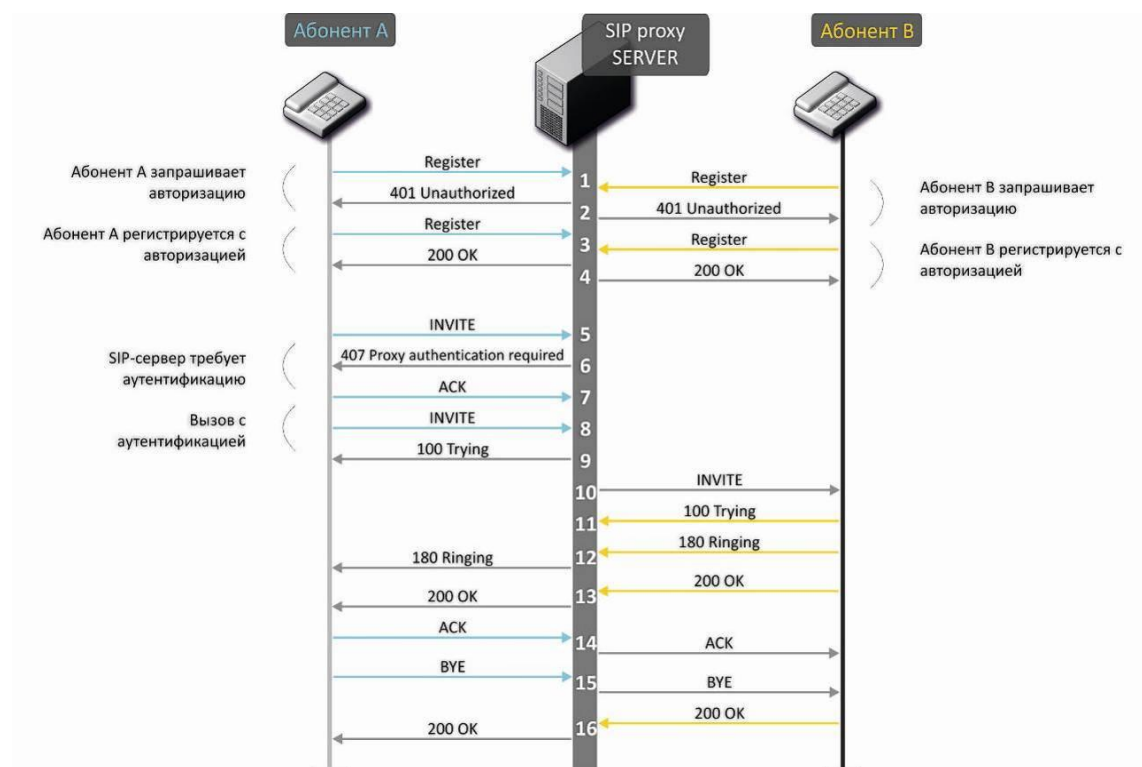
Рисунок 22 – Алгоритм вызова с участием SIP проху-сервера
