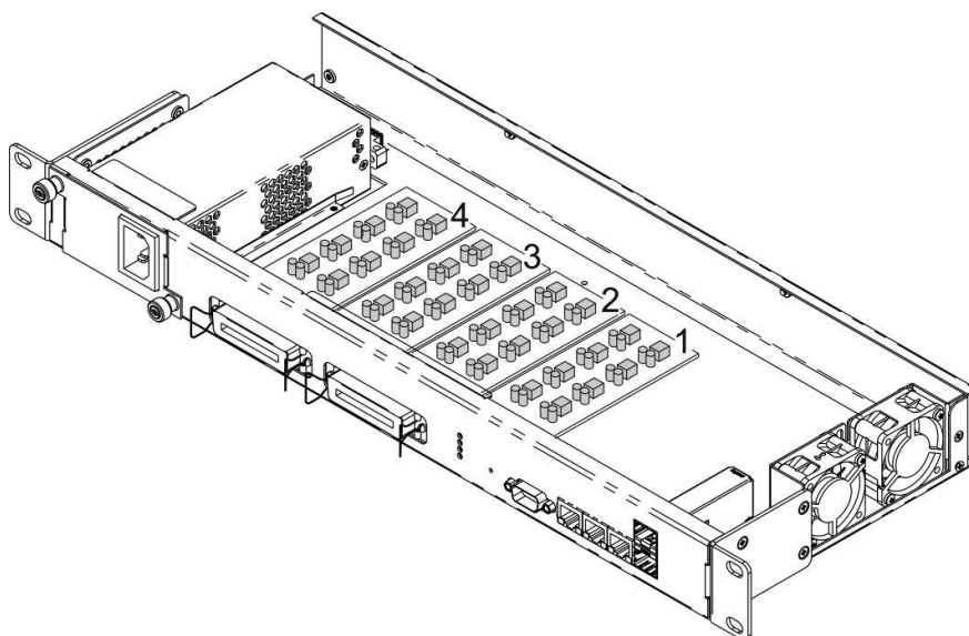
Рисунок 13 – Расположение субмодулей в TAU-32M.IP.
