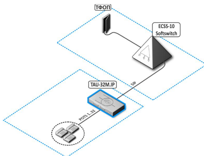
Рисунок 1 – Абонентский вынос TAU-32M.IP
