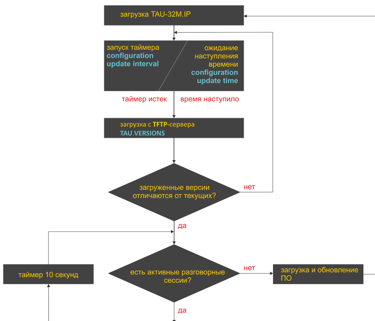
Рисунок 27 – Алгоритм работы функции автоматического обновления и проверки актуальности ПО
