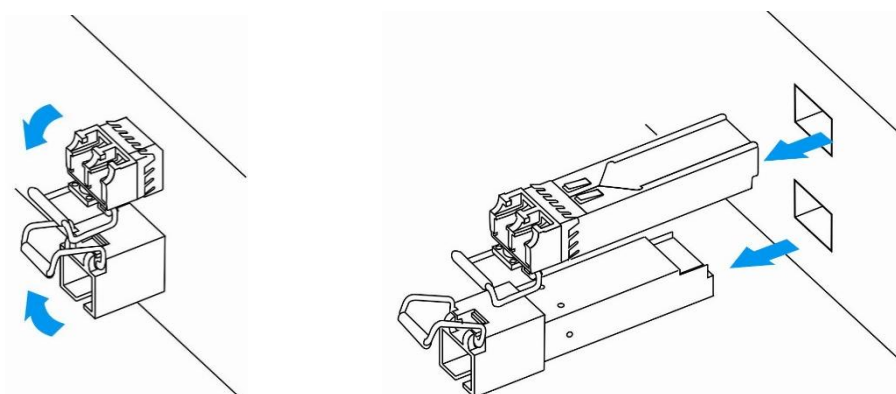
Рисунок 15 – Открытие защелки SFP-трансиверов и извлечение SFP-трансиверов
