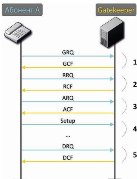
Рисунок 25 – Алгоритм вызова через гейткипер
