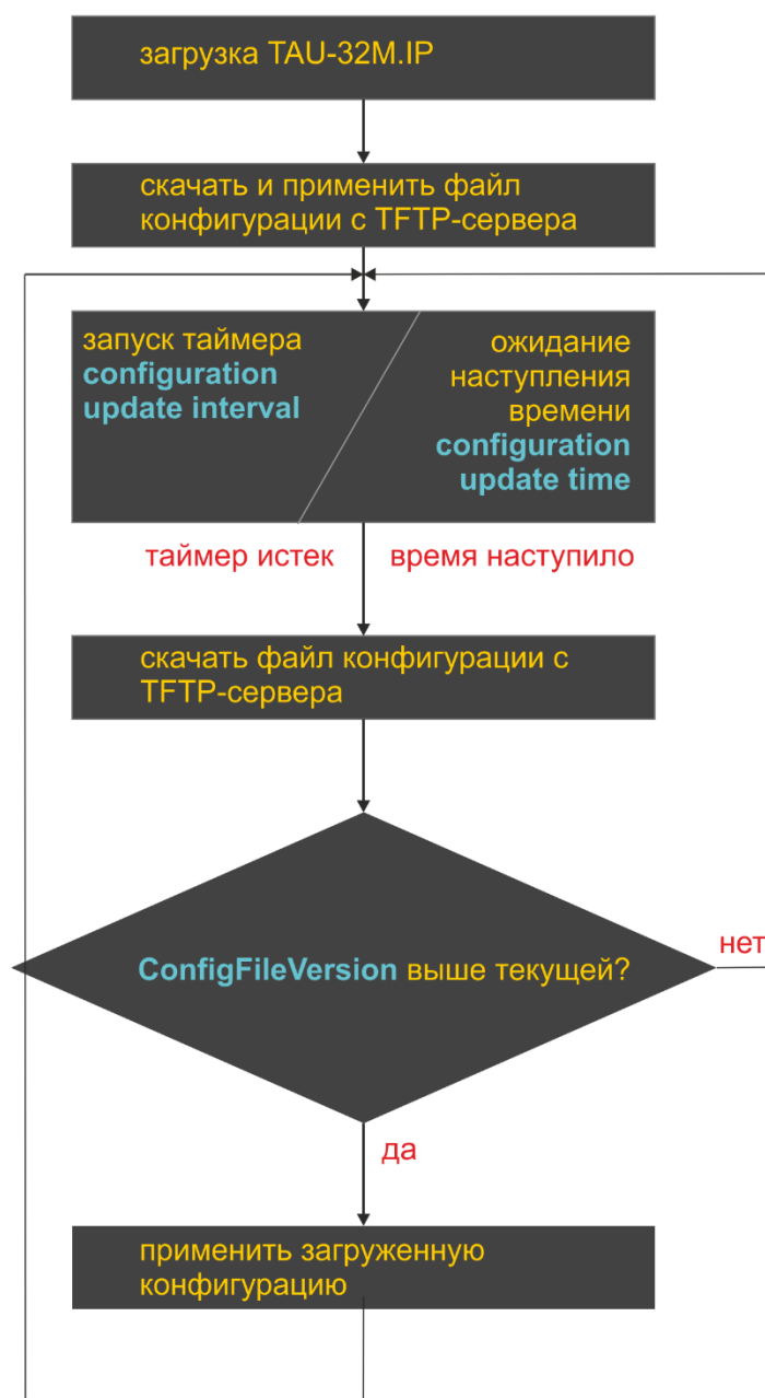
Рисунок 26 – Алгоритм работы функции автоматического конфигурирования TAU-32M.IP и проверки актуальности файла конфигурации
