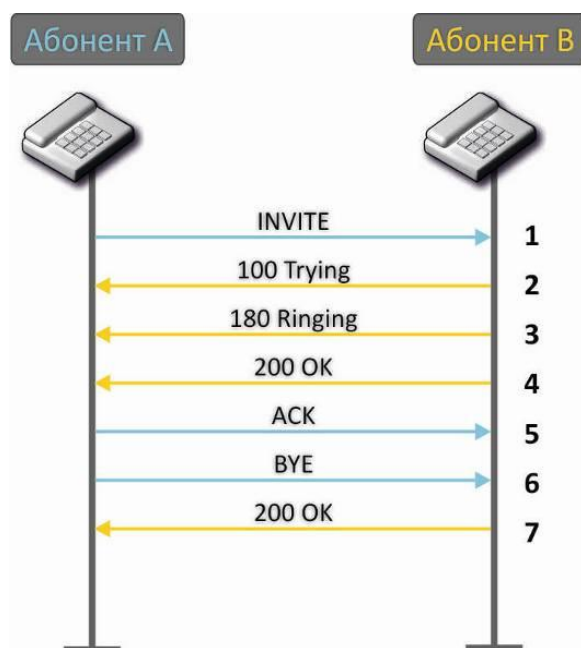
Рисунок 21 – Алгоритм вызова по протоколу SIP
