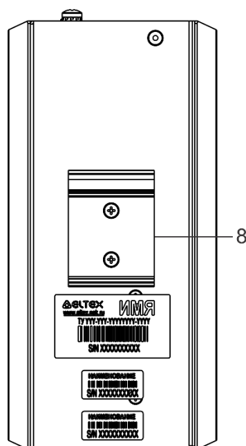
Рисунок 57 – Задняя панель MES3500I-08P, MES3500I-10P
