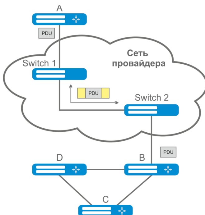
Рисунок 115 — Пример работы функции L2PT
