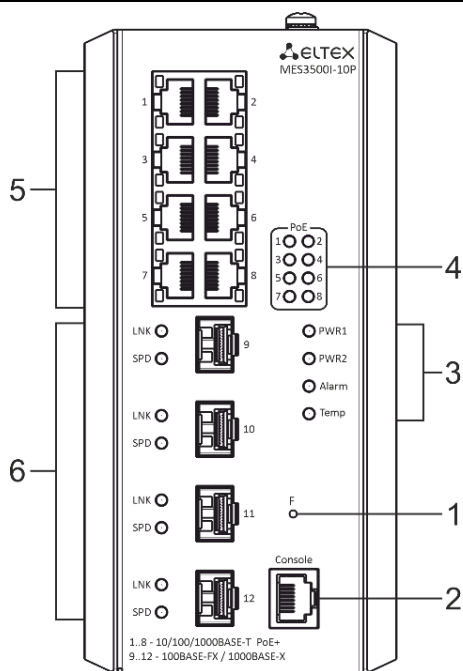
Рисунок 38 – Передняя панель MES3500I-10P
