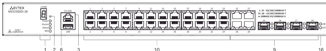
Рисунок 8 – Передняя панель MES2300DI-28
