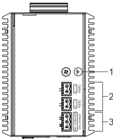
Рисунок 40 – Верхняя панель MES3500I-08P, MES3500I-10P
