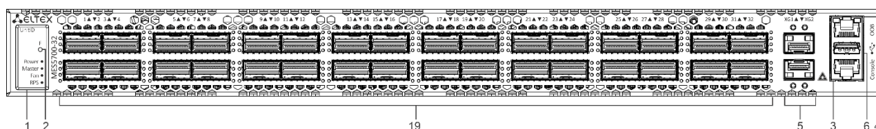
Рисунок 36 – Передняя панель MES5700-32
