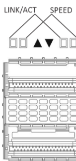
Рисунок 95 – Внешний вид разъема QSFP+ и QSFP28 для MES5300-48, MES5305-48, MES5310-48, MES5400-xx, MES5410-48
