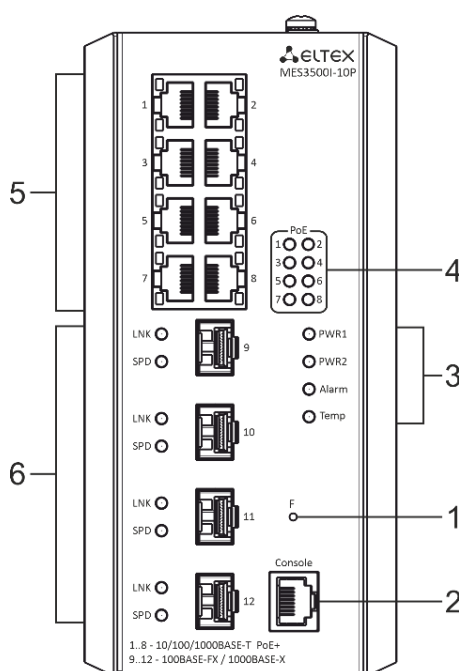
Рисунок 37 – Передняя панель MES3500I-08P
