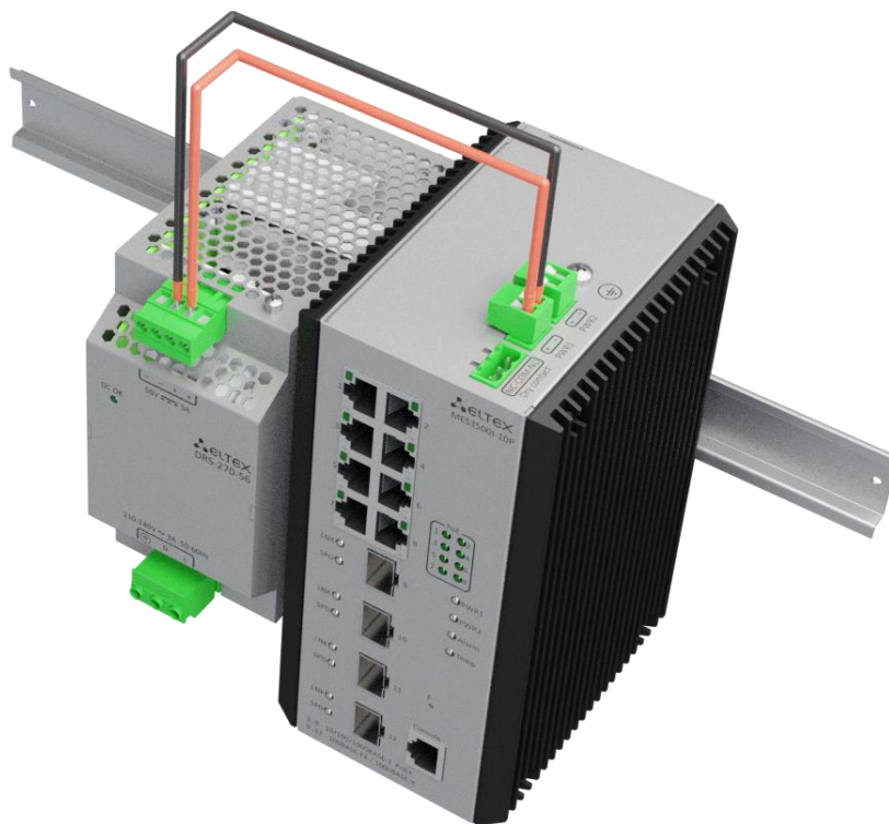
Рисунок 105 – Подключение питания коммутатора от DRS-270-56
