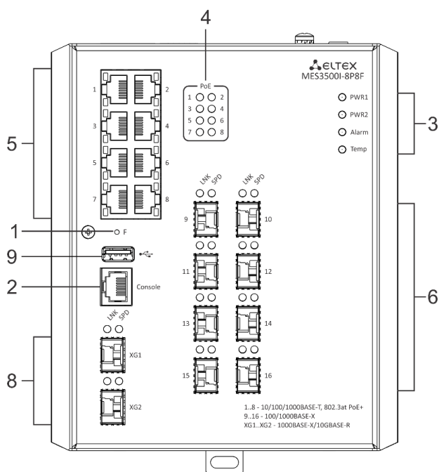
Рисунок 39 – Передняя панель MES3500I-8P8F
