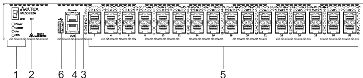
Рисунок 26 – Передняя панель MES5332A
