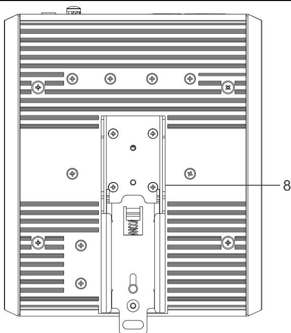
Рисунок 58 – Задняя панель MES3500I-8P8F
