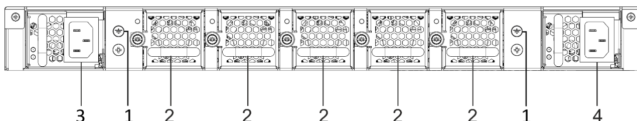
Рисунок 65 – Задняя панель MES5500-32
