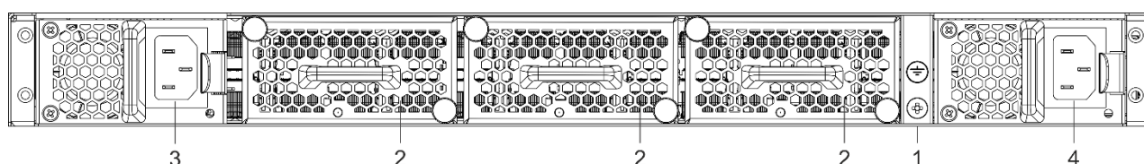
Рисунок 66 – Задняя панель MES5700-32
