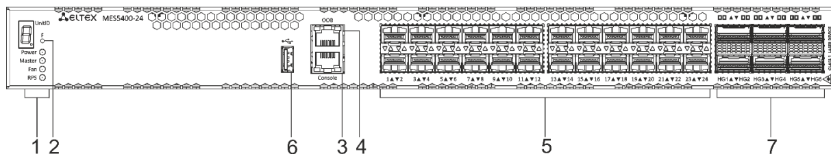
Рисунок 32 – Передняя панель MES5400-24
