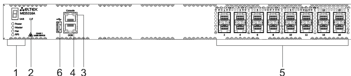
Рисунок 24 – Передняя панель MES5316A
