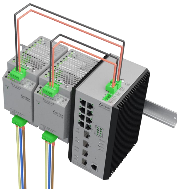
Рисунок 108 – Подключение промышленного коммутатора от двух блоков питания DRS-270-56
