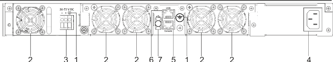
Рисунок 63 – Задняя панель MES5400-48
