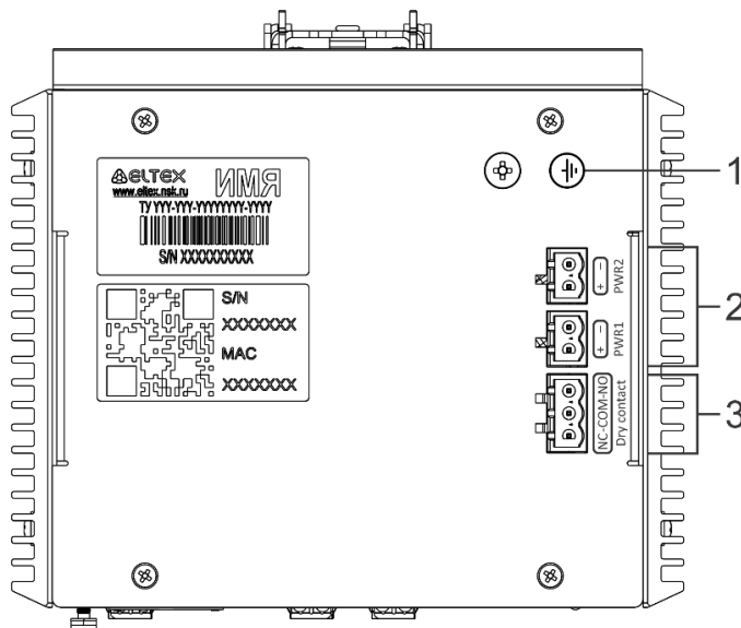
Рисунок 41 – Верхняя панель MES3500I-8P8F
