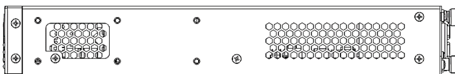
Рисунок 83 – Правая боковая панель MES5316A, MES5324A, MES5332A
