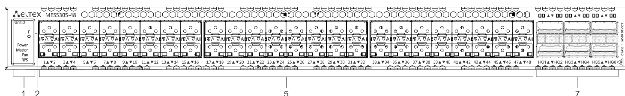
Рисунок 29 – Передняя панель MES5305-48
