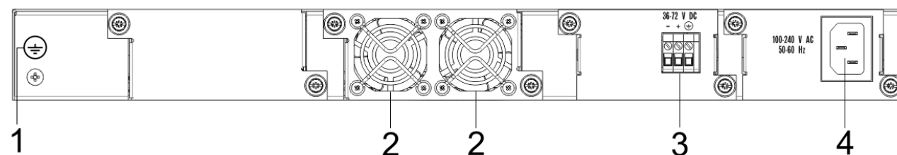
Рисунок 60 – Задняя панель MES5316A
