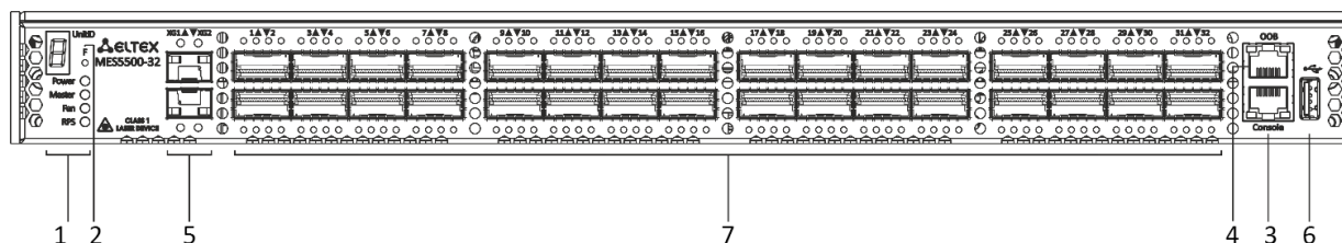
Рисунок 35 – Передняя панель MES5500-32
