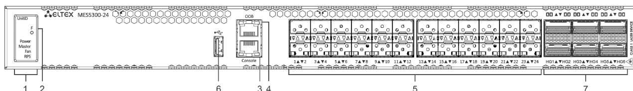
Рисунок 27 – Передняя панель MES5300-24
