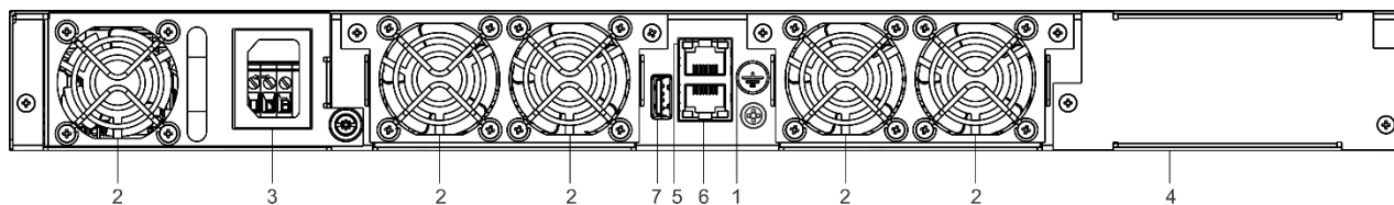
Рисунок 61 – Задняя панель MES5300-48, MES5305-48, MES5310-48
