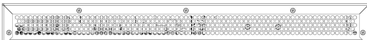
Рисунок 43 – Задняя панель MES2300-08P
