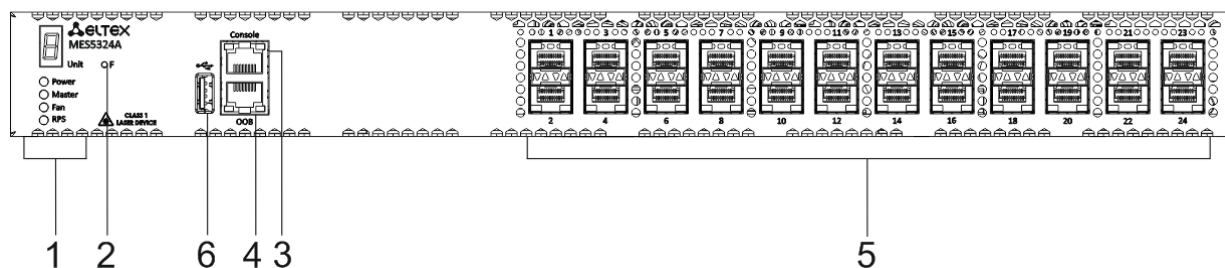
Рисунок 25 – Передняя панель MES5324A
