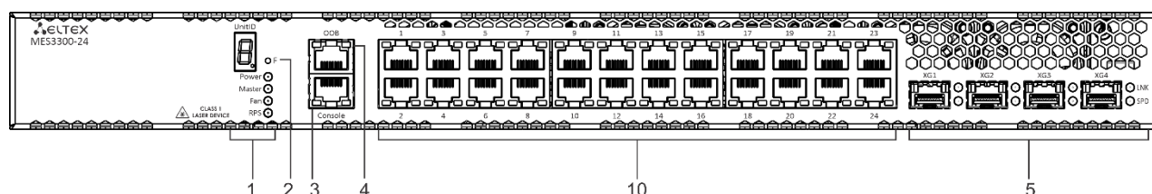
Рисунок 16 – Передняя панель MES3300-24
