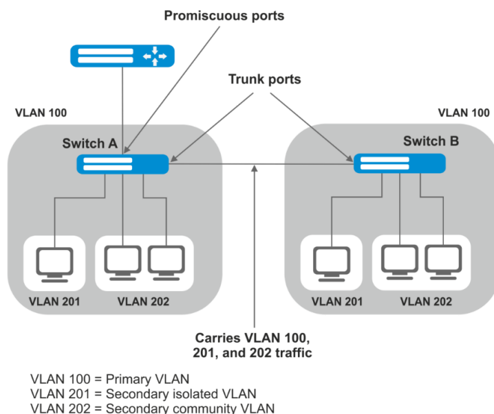
Рисунок 114 – Пример работы технологии Private VLAN
