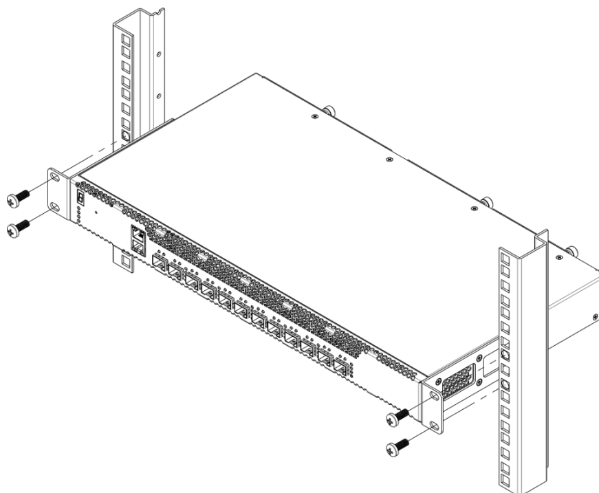
Рисунок 100 – Установка устройства в стойку
