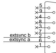
Разъем синхронизации
