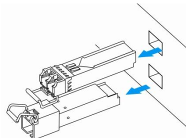
Рисунок 45 – Извлечение SFP-трансиверов
