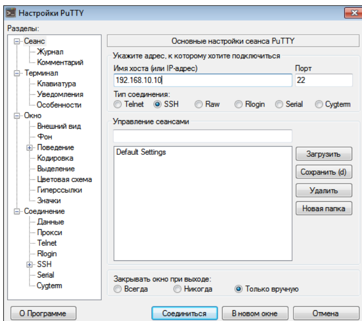
Рисунок 2 – Запуск SSH-клиента
