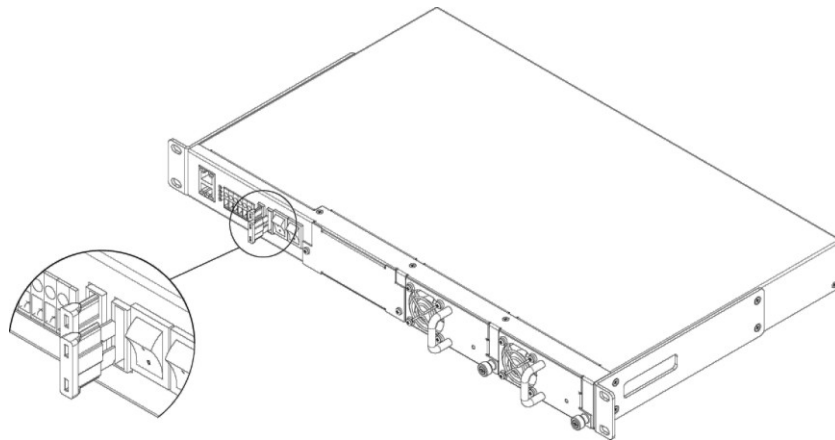
Рисунок 8 – Замена предохранителей
