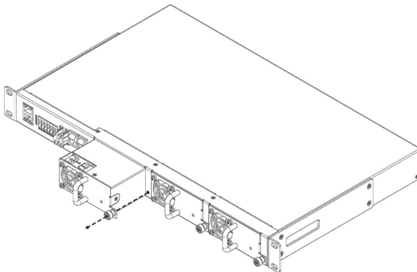
Рисунок 6 – Снятие заглушки
