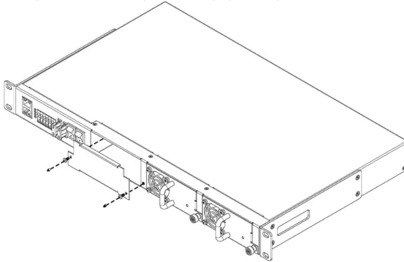
Рисунок 6 – Снятие заглушки
