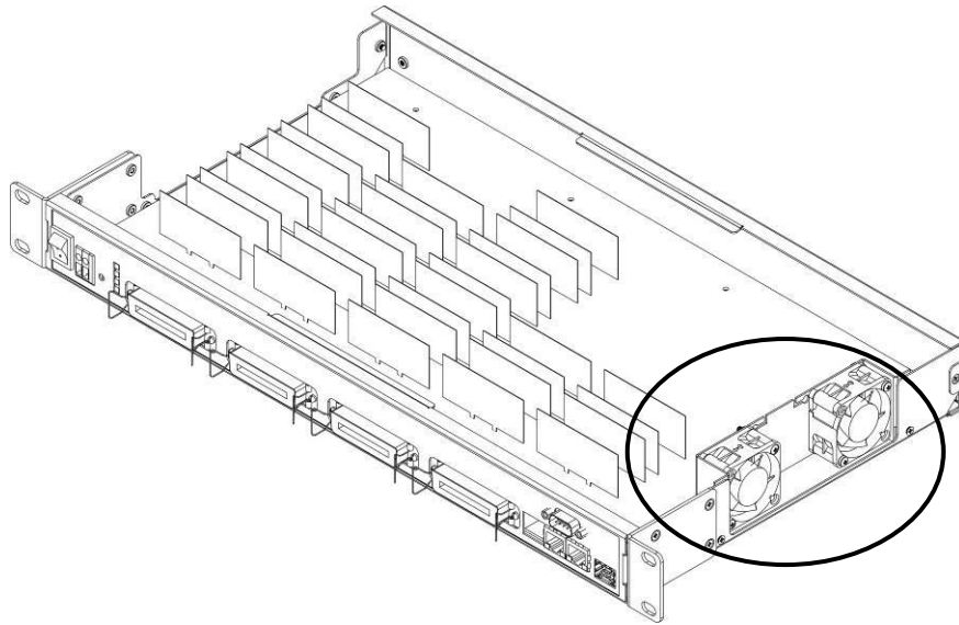
Fig. 6 - Fan location
