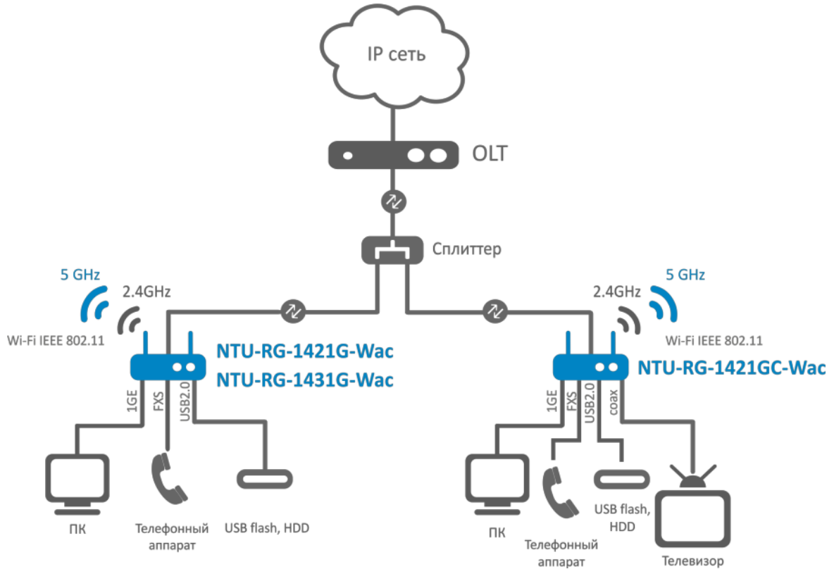
Рисунок 1 – Схема применения NTU-RG-1421G-Wac, NTU-RG-1431G-Wac, NTU-RG-1421GC-Wac
