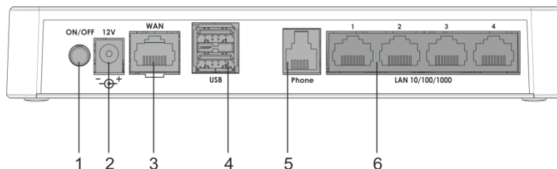
Рисунок 5 – Внешний вид задней панели RG-5421G-Wac
