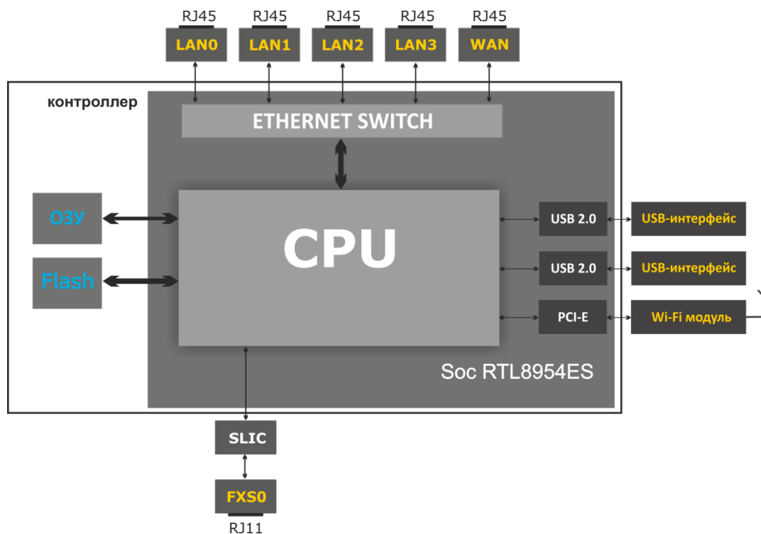
Рисунок 2 – Структурная схема RG-5421G-Wac
