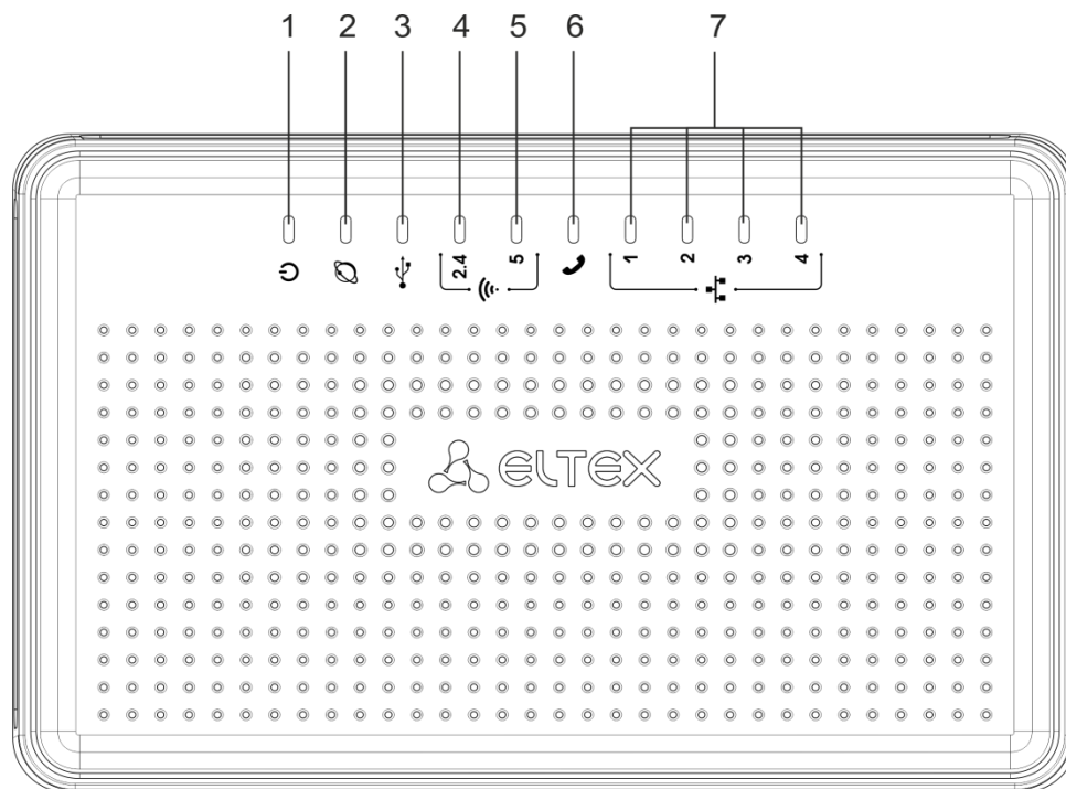
Рисунок 4 – Внешний вид передней панели RG-5421G-Wac
