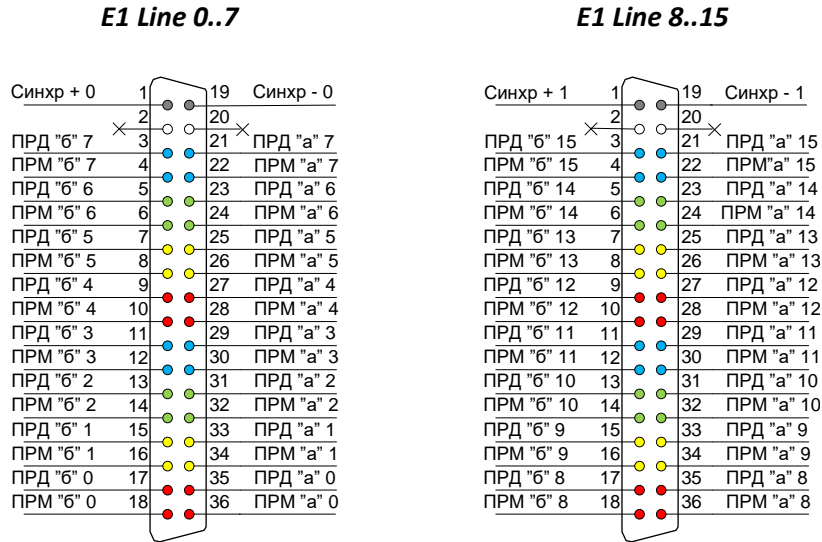
Рисунок 39 – Назначение контактов разъемов E1 Line
