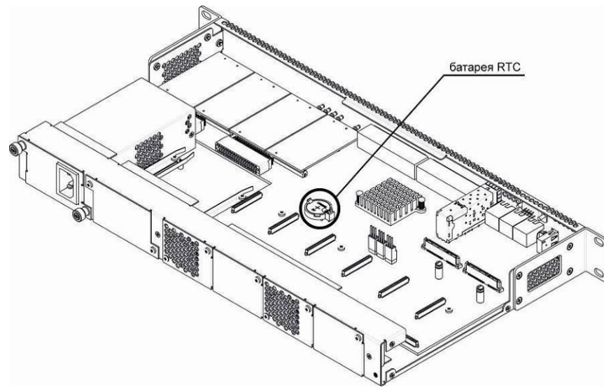
Рисунок 32 – Положение батареи RTC для SMG-1016M
