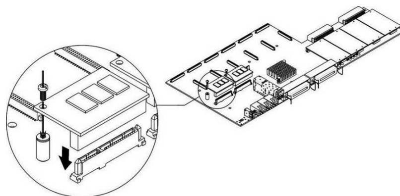
Рисунок 28 – Монтаж SSD-накопителя
