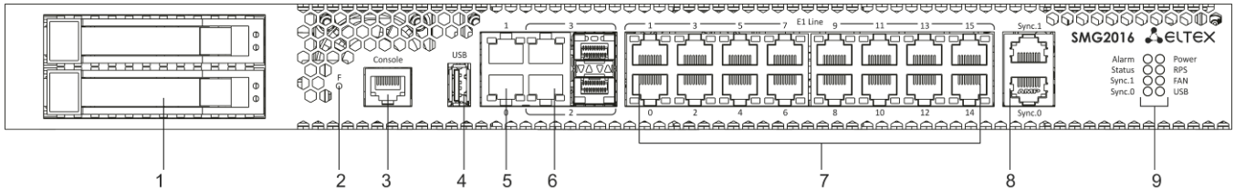
Рисунок 12 – Внешний вид передней панели SMG-2016
