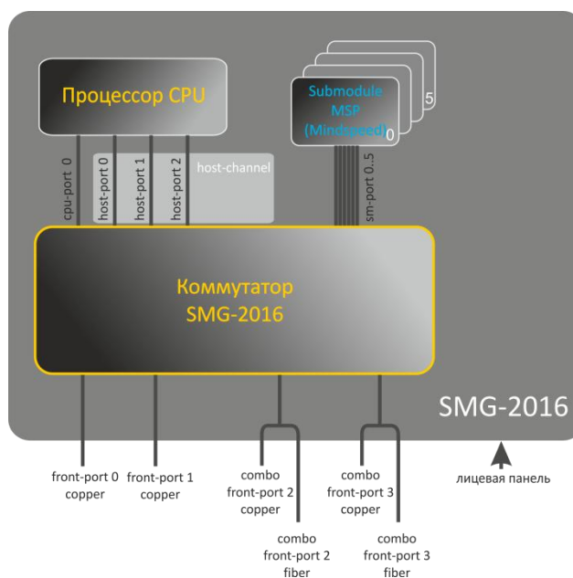
Рисунок 38 – Структура коммутатора
