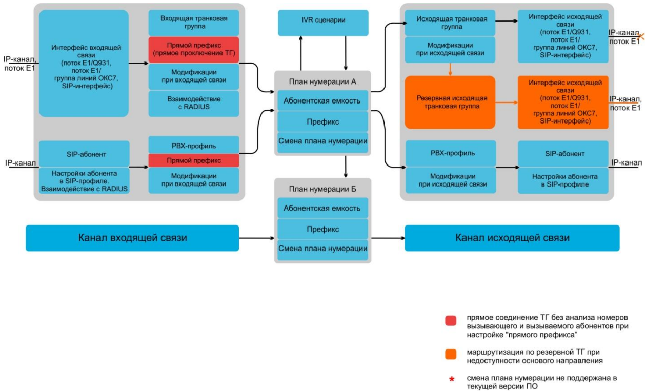
Рисунок 43 – Взаимосвязь параметров маршрутизации, абонентов и СЛ
