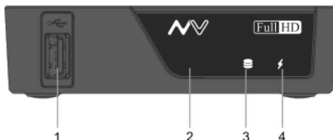
Рисунок 2 – Внешний вид передней панели STB NV-100/NV-102
