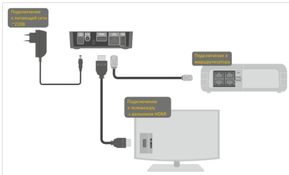
Рисунок 11 – Пример подключения медицентра NV-100/NV-102
